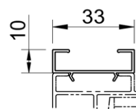
en option: cale de rattrapage 10mm P x 33mm L
