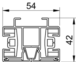
glissière ZIP couplée 42mm P x 54mm L
